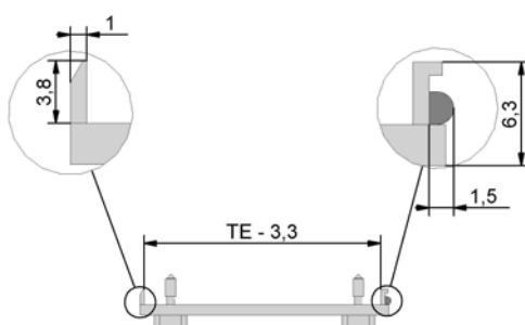
Вид сверху, U-образный профиль
