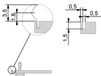
Вид сверху, Future
