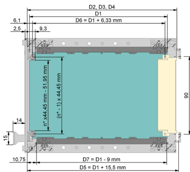
Вид сбоку, стандартная модель
