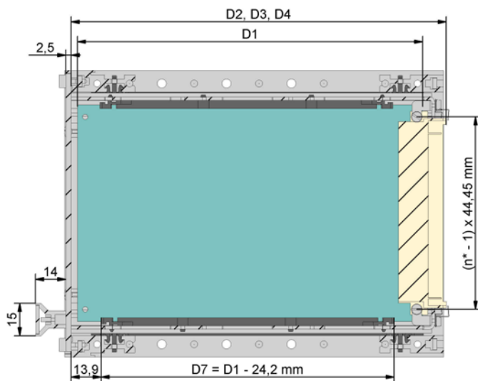
Вид сбоку, кассеты, экранированные
