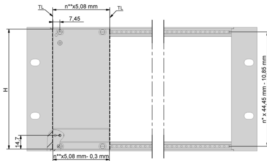
Монтажные размеры (мм)
