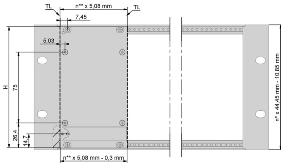
Главный вид сменного модуля, стандартная модель
