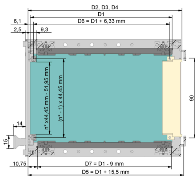
Размеры для вставных модулей (мм)
